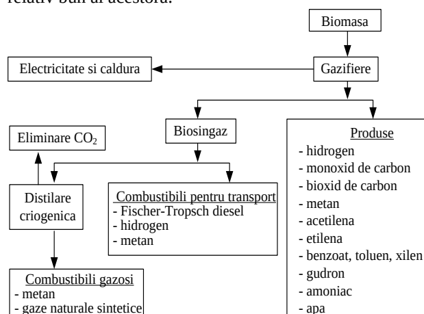
Figura 2. Derivate ale singazului produs din biomasa solidă
