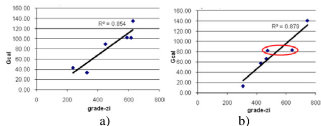
Fig. 2. Corelația dintre consumul lunar de energie și HDD pe sezonul termic, 2010-2011 (a) și 2011-2012 (b).
