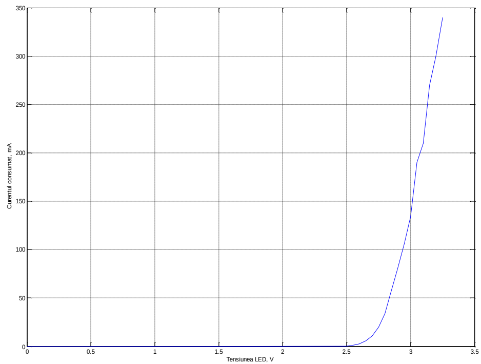
Fig.5. Caracteristica de putere a LED-ului
