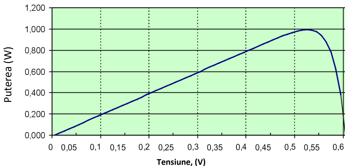
Fig.2. Caracteristica de putere a celulei fotovoltaice
