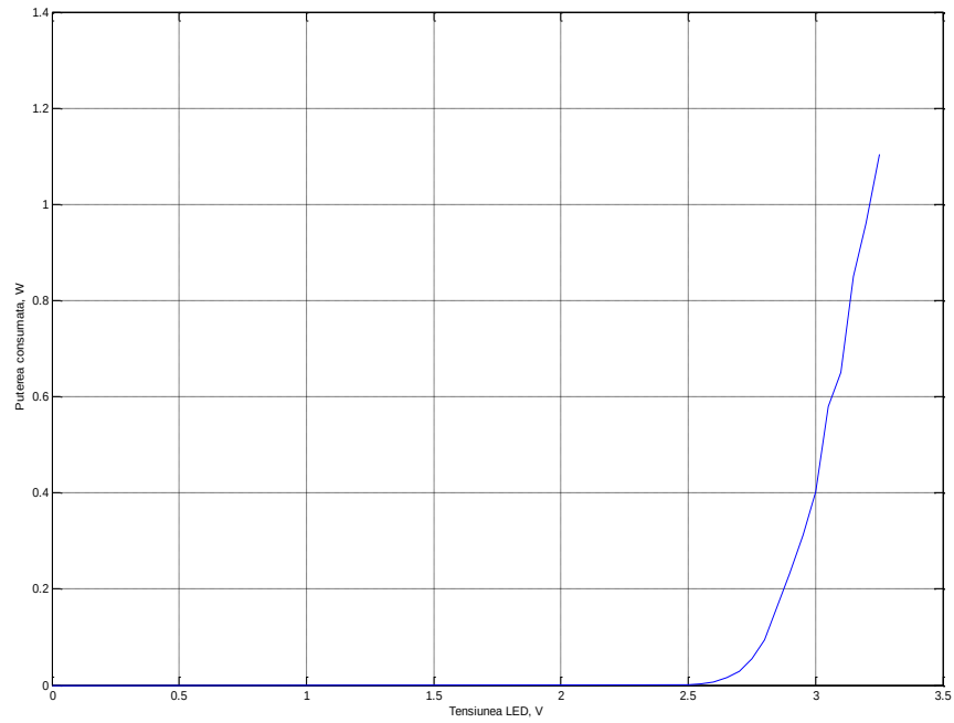
Fig.4. Caracteristica tensiune – curent a LED-ului
