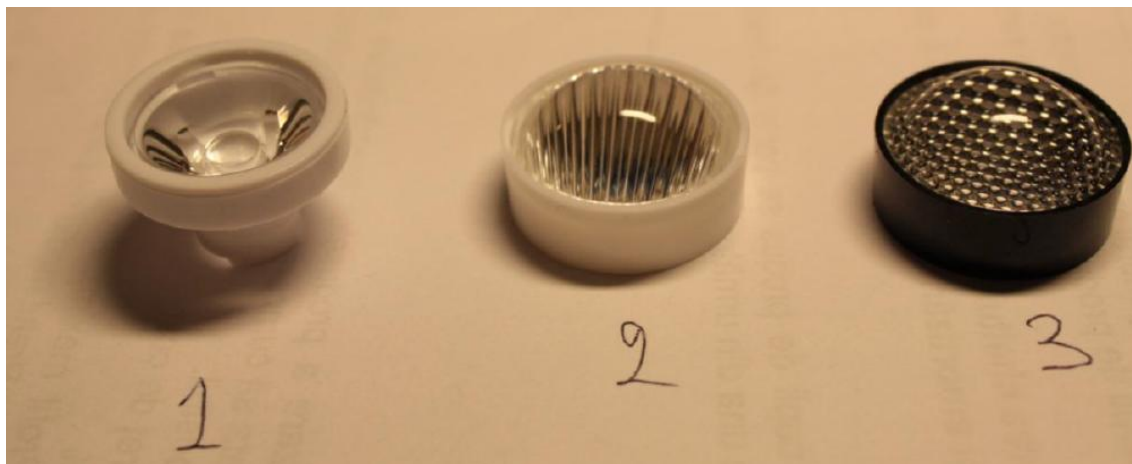
Fig.6. Tipuri de dispersatoare cercetate
